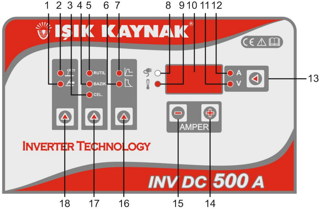
Şekil 3: Kontrol Paneli
